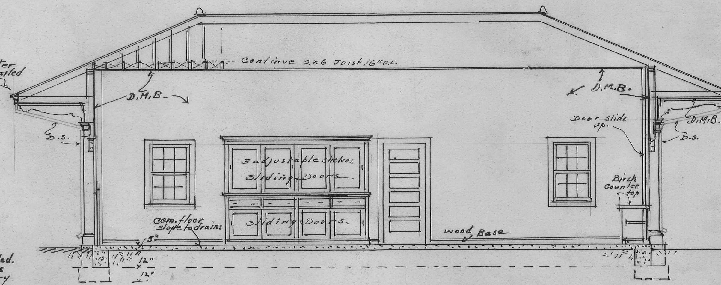
LONGITUDINAL SECTION
